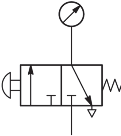
Abbildung 3: Schaltschema
