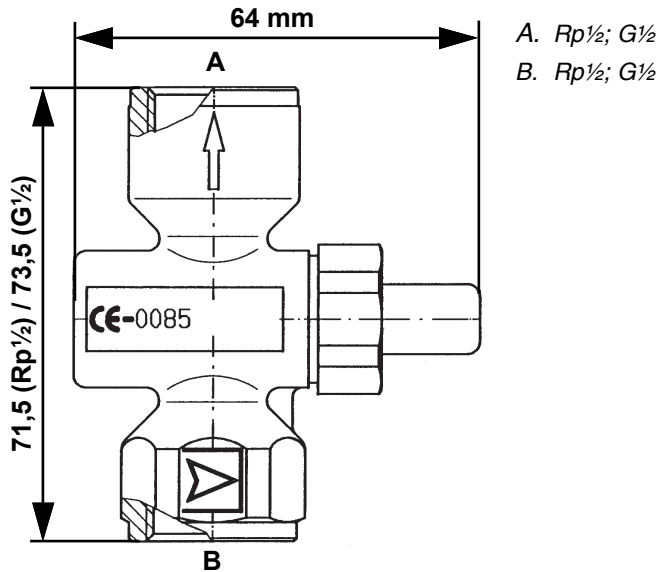
Abbildung 1: Abmessungen und Anschlüsse (Rp 1/2; G 1/2)
