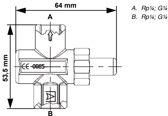
Abbildung 2: Abmessungen und Anschlüsse (Rp 1/4; G 1/4)
