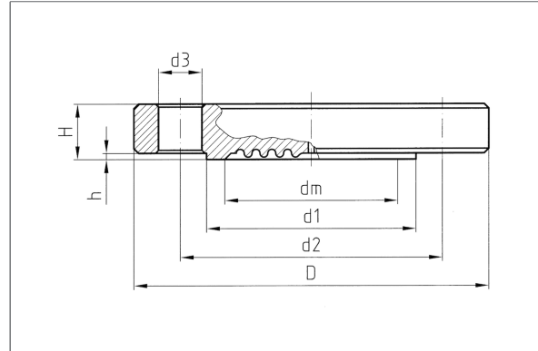
Typ MD 80 - Flanschanschluss nach EN 1092-1 Form B 1
