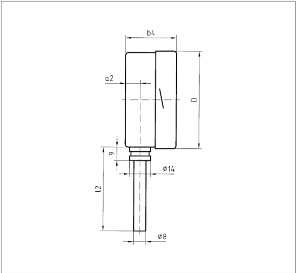
Maße (mm)
