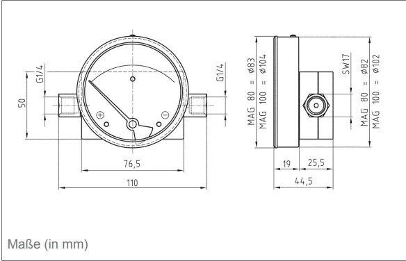
Anschluss rechts und links, seitlich
